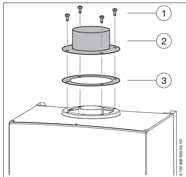
Рис. 18 Крепление переходника
