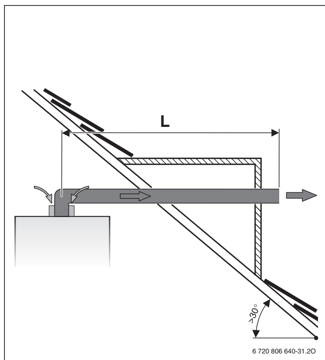
Рис. 6 Горизонтальный отвод дымовых газов B 22
