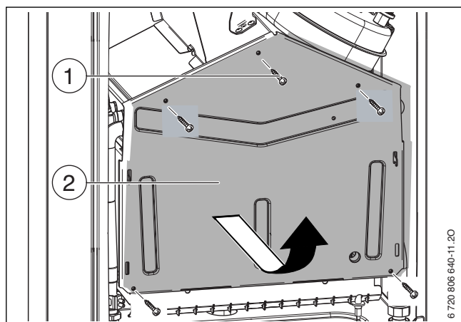
Рис. 39 Открытие горелки
