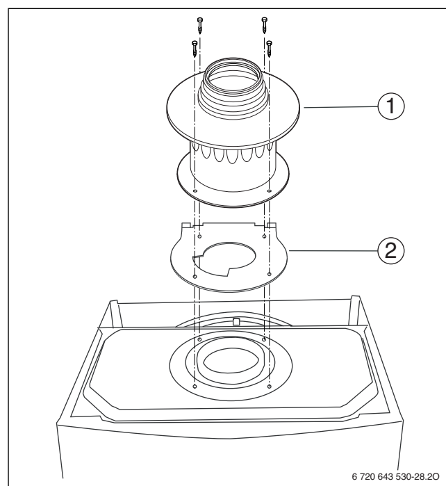
Рис. 19 Установка переходника в системе отвода дымовых газов В 22 и при наличии дроссельной диафрагмы
