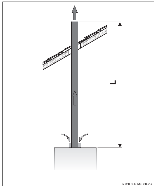
Рис. 7 Вертикальный отвод дымовых газов B 22
