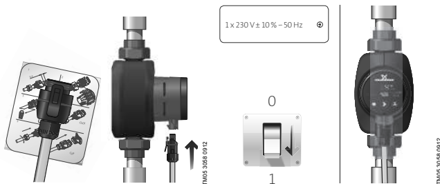
10-сур. Электр желісіне қосу
