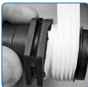
Намотка фум-ленты
