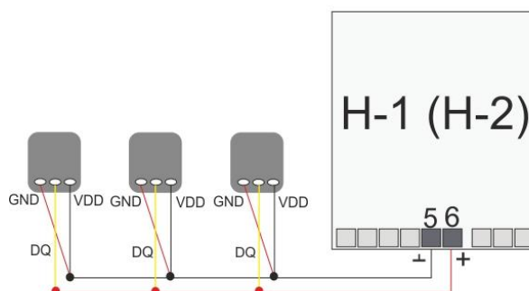
Датчик DS18B20
